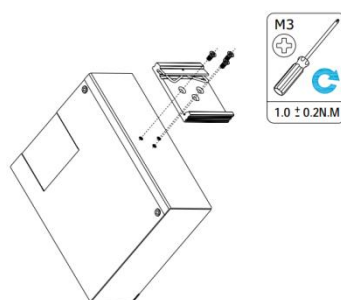
DIN 导轨安装
