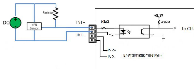
DI 连接示意图
