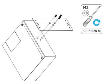
壁挂式安装
